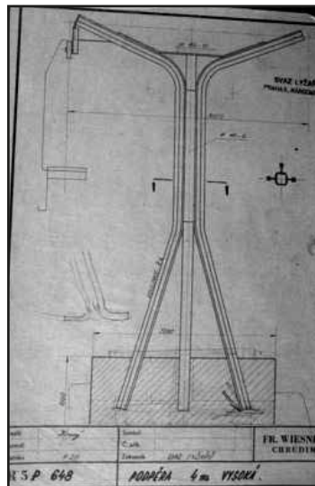
Nákres podpěry lanového výtahu
