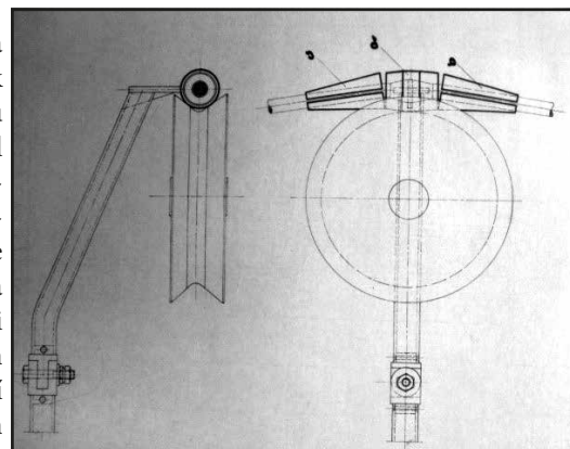
Nákres závěsu sedačky
